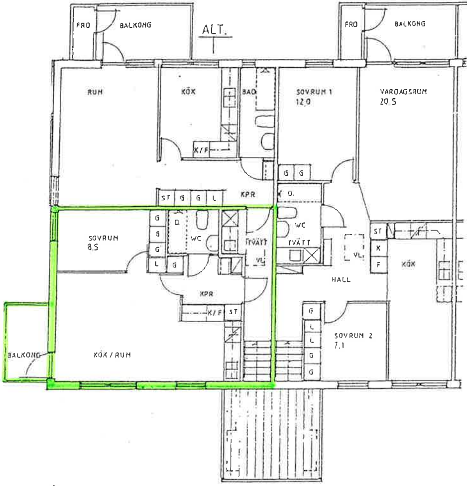
VÅN 1 TRP
